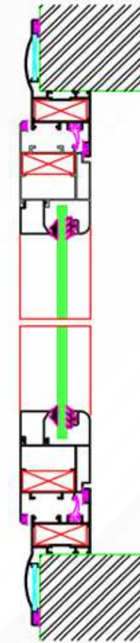
SECTION A-A
