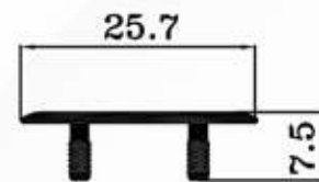
EG 9609 0.154 Kg/ml.
