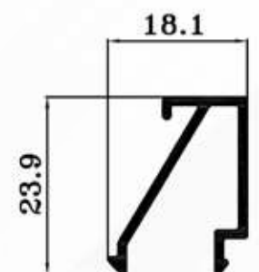
EG4813 0.194 Kg/ml.
