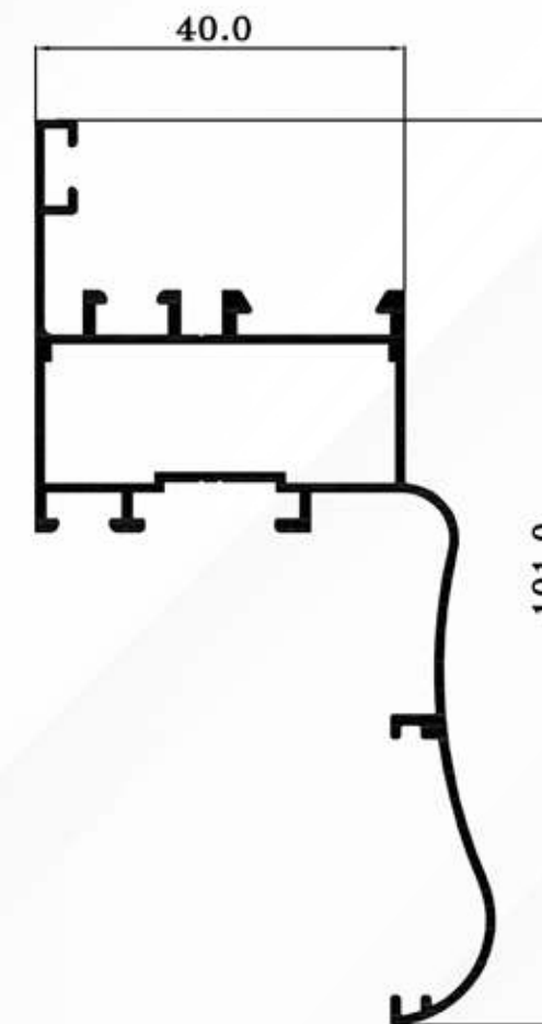
EG4862 Kg/ml.
