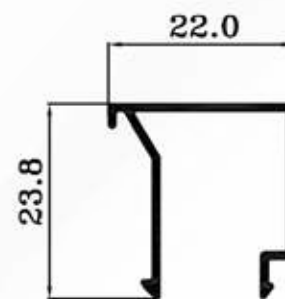
EG4811 0.224 Kg/ml.
