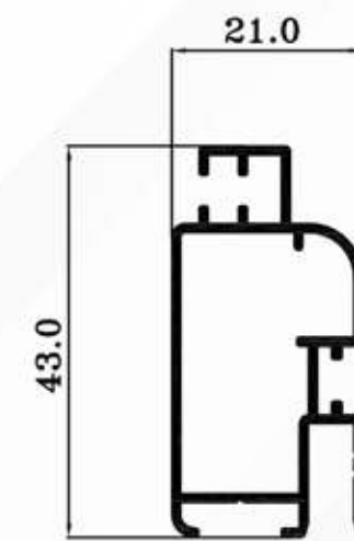
EG 6606 0.500 Kg/ml.
