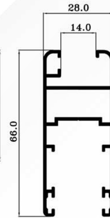
EG 6602 0.780 Kg/ml.
