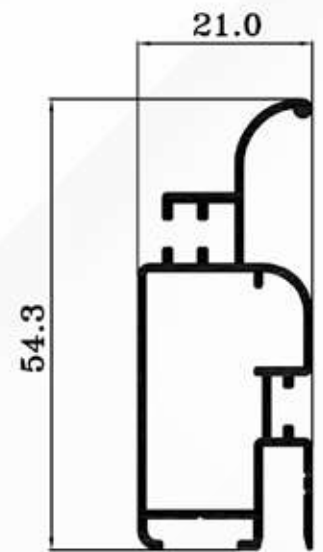
EG 6006 0.570 Kg/ml.
