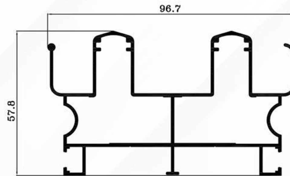
EG 9601 1.540 Kg/ml.
